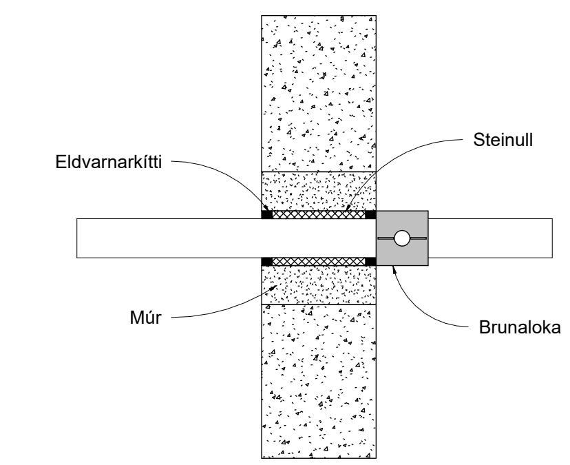
Brunapétting á loftræstilögn í gegnum steypnan vegg
