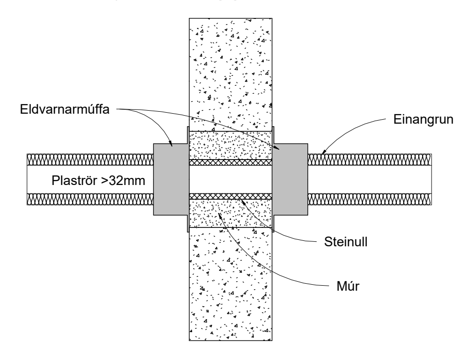
Brunapétting á plastlögn stærri en Ø32mm í gegnum steypnan vegg
