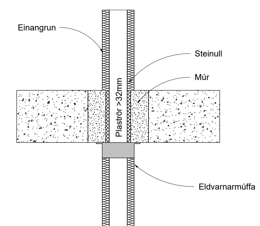
Brunapétting á plastlögn stærri en Ø32mm í gegnum steypnt gólf
