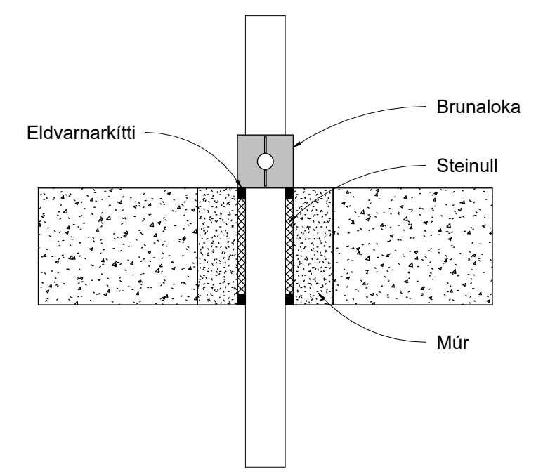
Brunapétting á loftræstilögn í gegnum steypnt gólf utan lagnaskakts
