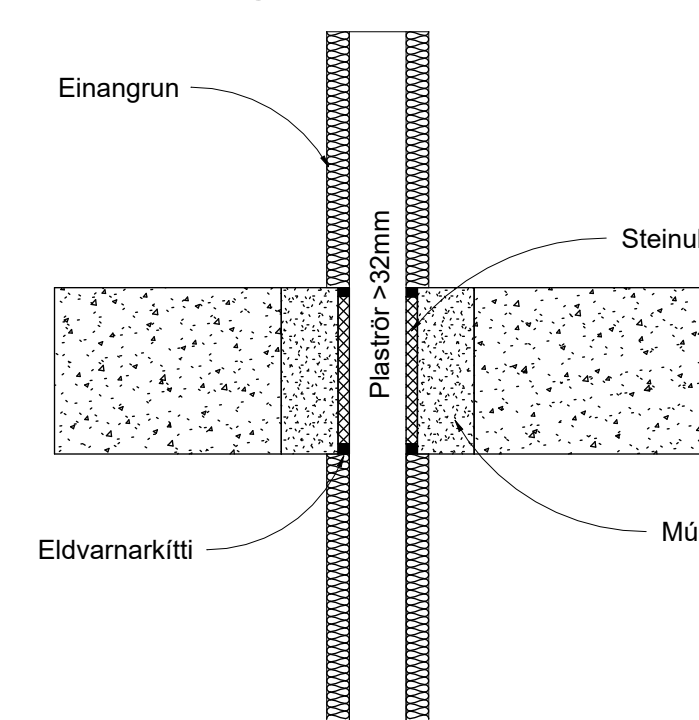
Brunapétting á plastlögn stærri en Ø32mm í gegnum steypnt gólf innan lagnaskakts
